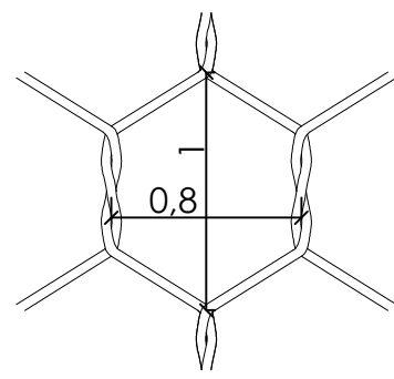
Dettaglio maglia gabbionata
